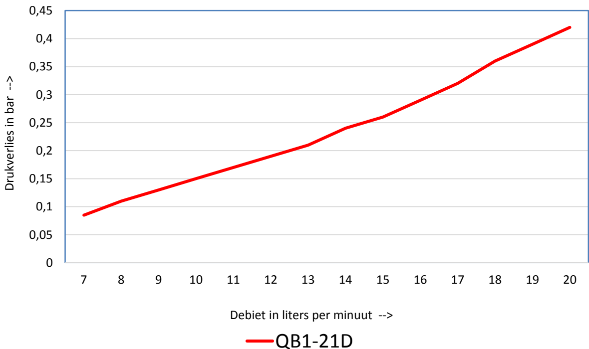
Grafiek drukval Showersave® QB1-21D
